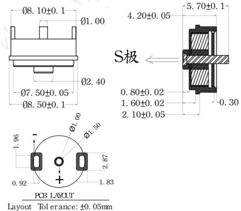
cx-8.3mm-F 3A 12V
