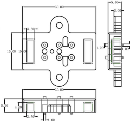
双排6pin公
