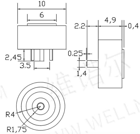
cx 908B-8-10mm-F 磁铁Φ8 塑料Φ10 3A 12V
