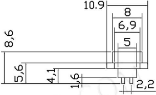
CXZ-D型-17pin公
