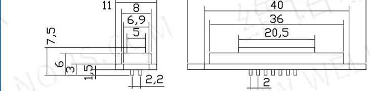
CXZ-D型-13pin母
