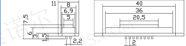
CXZ-D型-14pin母
