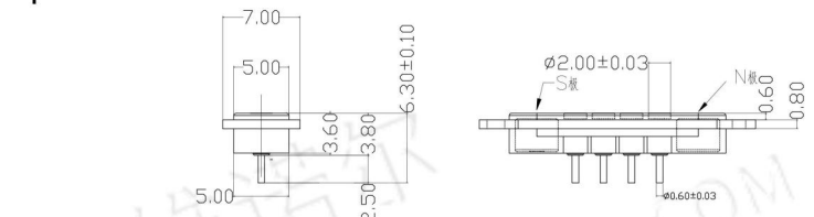
4p-2.54PH-02
