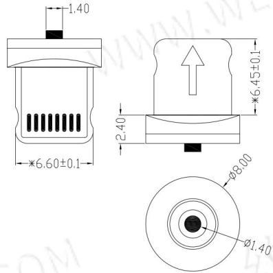
cx-3mm-M 长脚 超薄磁吸 3A 12V
