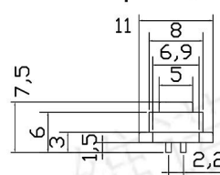
CXZ-D型-19pin母
