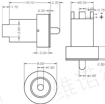
cx-902-8mm 3A 12V
