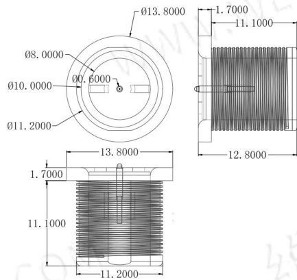
cx-11m-dc 螺纹Φ11防短路 3A 12V
