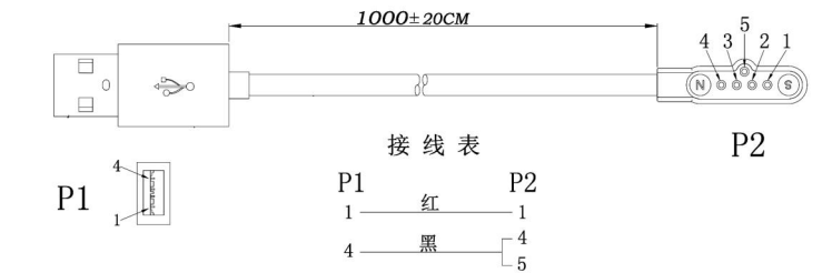
5pin-usb
