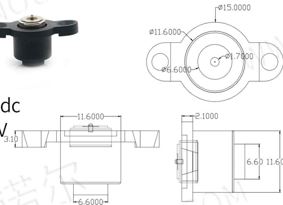
cx-15a-dc 螺纹Φ8磁吸 3A 12V
