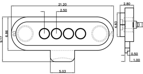
B型4pin贴片母
