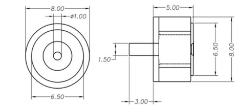
cx-907-8mm 黄铜
