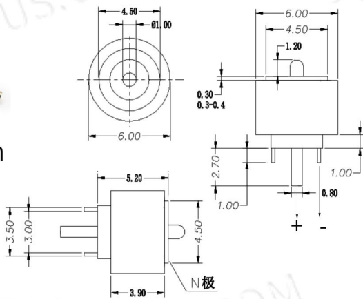
cx-902-6mm 3A 12V
