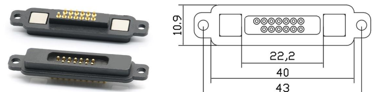
CXZ-D型-13pin公
