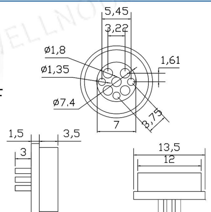
cx12-13.5mm-5P-F 2A 12V
