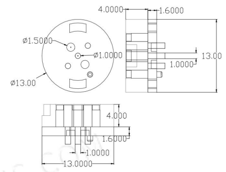
cx13mm-3P-F
