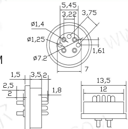
cx12-13.5mm-4P-F 2A 12V
