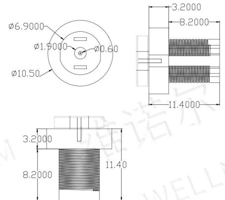
cx-08m-dc 螺纹Φ8防短路 3A 12V
