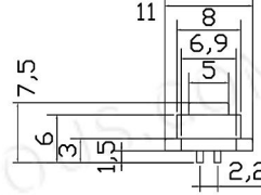
CXZ-D型-17pin母
