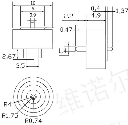
cx 908B-8-10mm-M 磁铁Φ8 塑料Φ10 3A 12V
