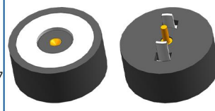
cx 908B-10-12mm-F 磁铁Φ10 塑料Φ12 3A 12V
