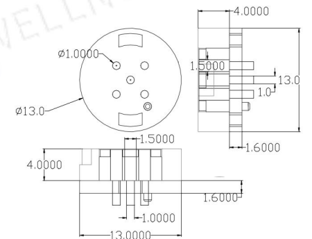
cx13mm-5P-F
