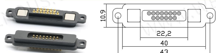
CXZ-D型-14pin公
