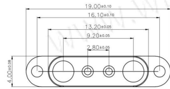
2p-2.84PH-02e
