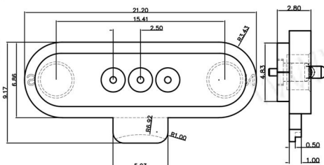
B型3pin插件母
