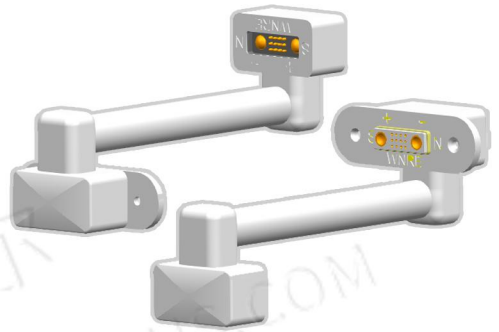
CX-2+12P公转母弯式
