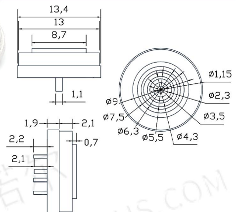
CX-MX4P-F
