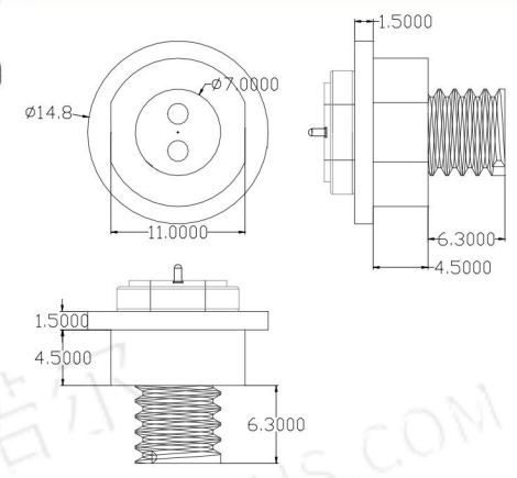
cx-15a-dc 螺纹Φ8磁吸 3A 12V
