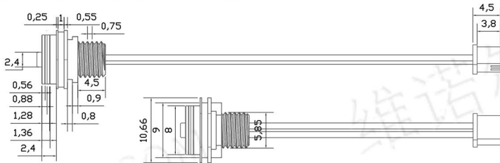
cx-06m-dc母带ZH端子
