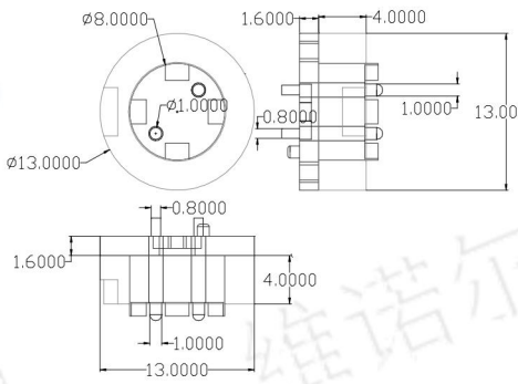
cx13mm-2P-M
