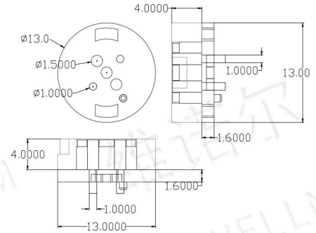
cx13mm-2P-F
