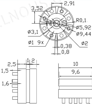
CX-A12mm-5P-M 2A 12V
