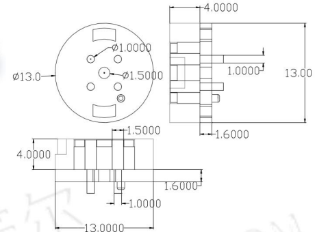
cx13mm-4P-F
