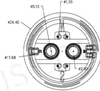
cxfs-27mmjg-f2 焊线 18A 24V
