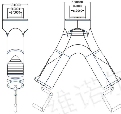
cx-10mm双勾线
