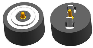
cx 908B-8-10mm-M 磁铁Φ8 塑料Φ10 3A 12V
