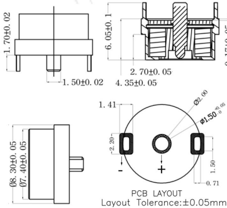
cx-8.3mm-M 防短路 3A 12V
