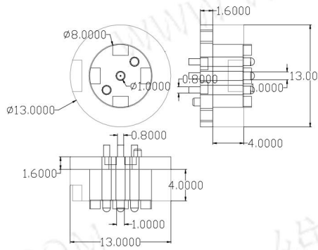
cx13mm-3P-F
