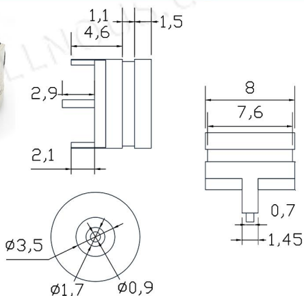
CX-CNC8-M 防短路
