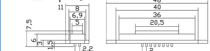
CXZ-D型-16pin母
