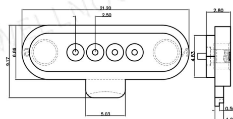
B型4pin插件母
