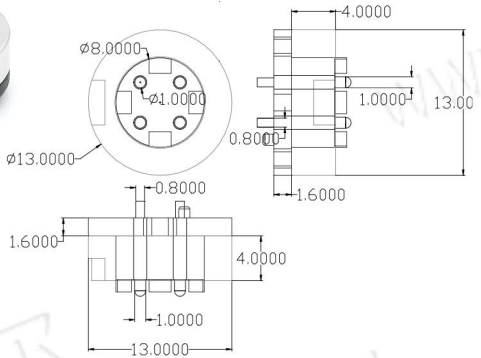
cx13mm-4P-M
