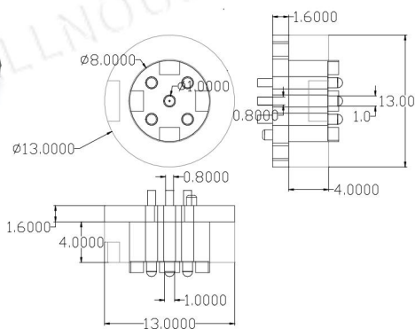
cx13mm-5P-M
