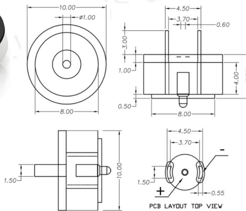
cx-908-10mm 3A 12V
