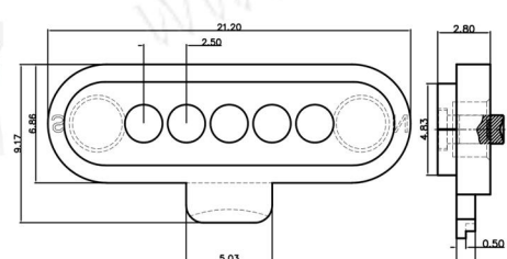
B型5pin贴片母
