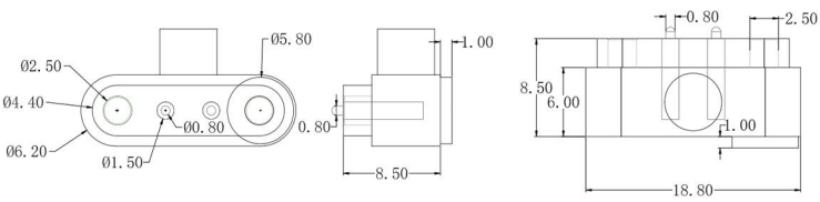
2pT-2.54PHT-usb
