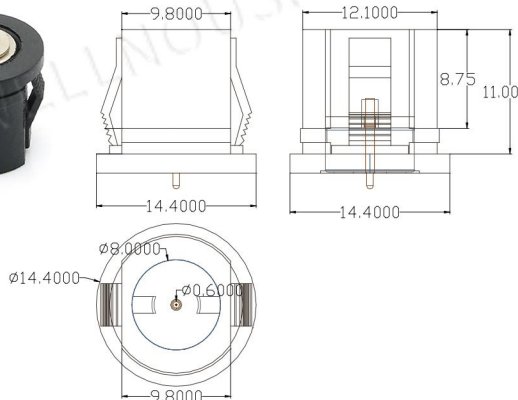
cx-12a-dc 卡扣磁吸 3A 12V
