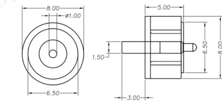
cx-906-8mm 黄铜
