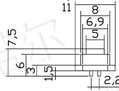
CXZ-D型-18pin母
