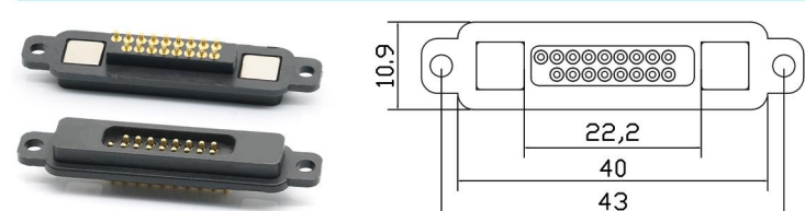
CXZ-D型-17pin公
