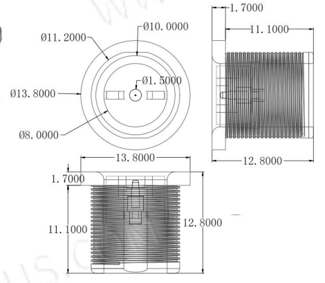
cx-11m-dc 螺纹Φ11防短路 3A 12V
